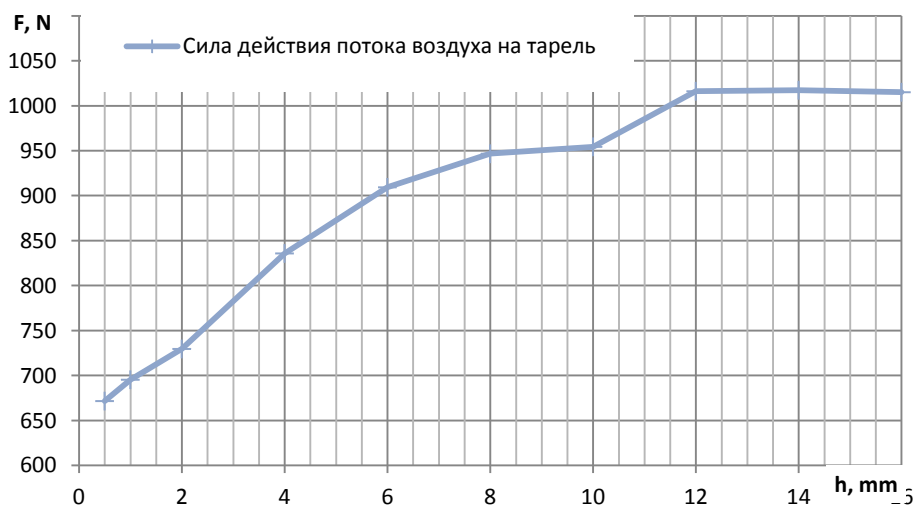
Рис. 4. Результат расчета аэродинамической силы действующей на тарель клапана
