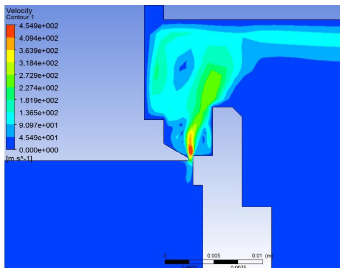
Рис. 7. Контур распределения скоростей ( h=0,5 мм) для геометрии с уступом глубиной 2 мм
