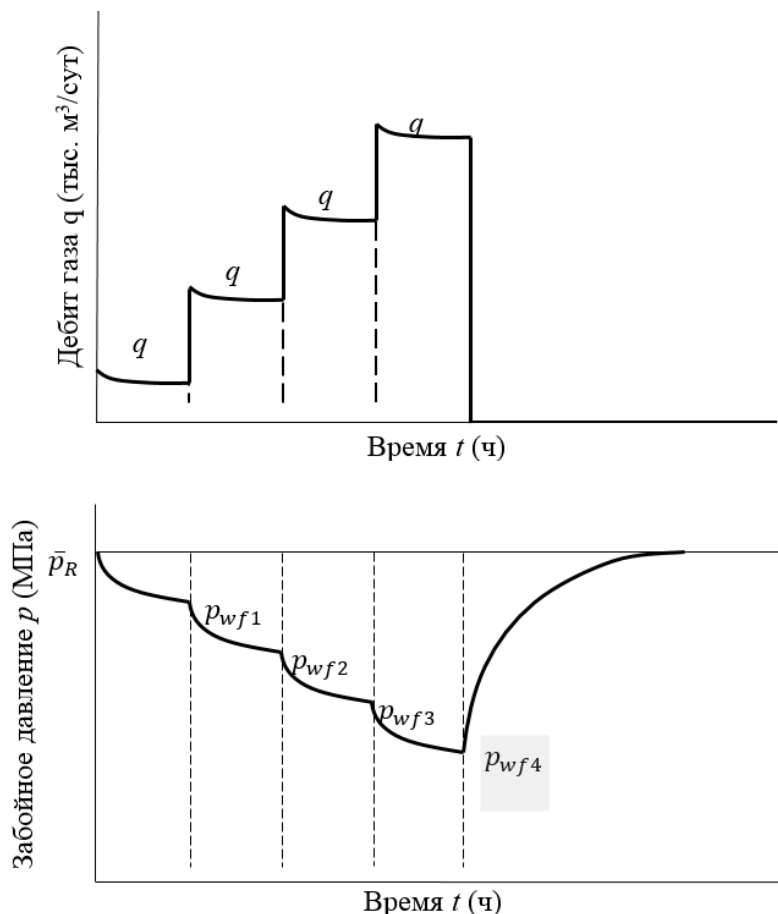
Рис. 1. Динамика изменения давлений и дебитов в ходе типового исследования газовой скважины на различных режимах работы
