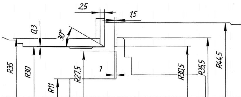
Рис. 10. Геометрия с уступом глубиной 1,5 мм
