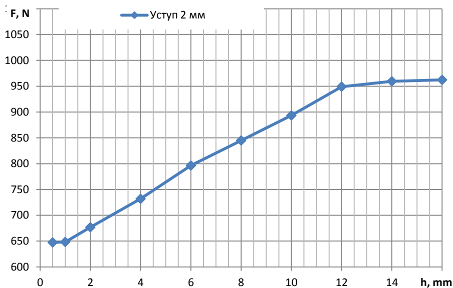
Рис. 6. Подъемная сила для клапана с уступом глубиной 2 мм
