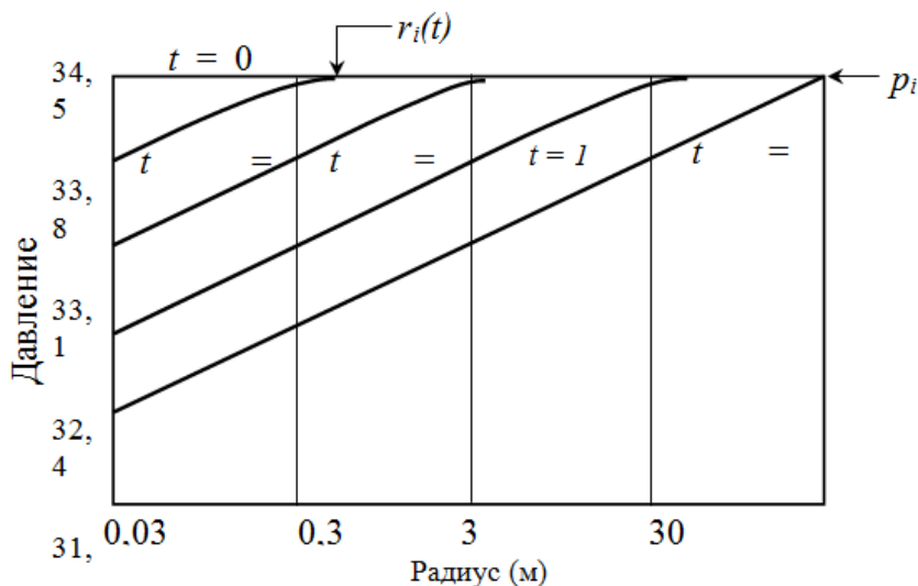
Рис. 1. Величина радиуса влияния в зависимости от продолжительности периода притока
