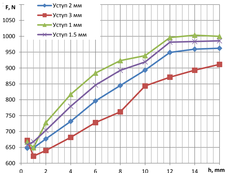
Рис. 12. Результаты моделирования тарелей с различной глубиной уступа
