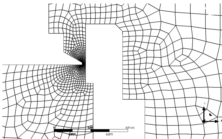
Рис. 3. Расчетная сетка
