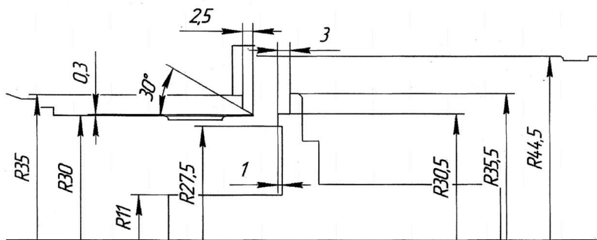
Рис. 11. Геометрия с уступом глубиной 3 мм
