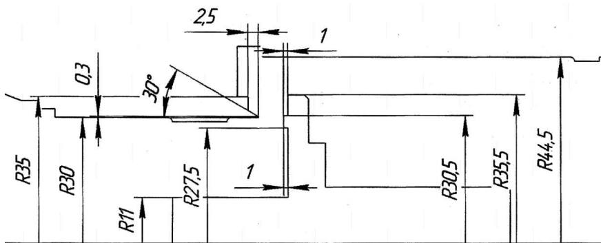
Рис. 9. Геометрия с уступом глубиной 1 мм
