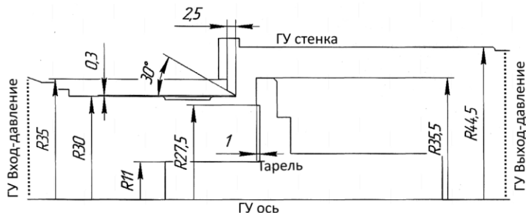
Рис. 2. Двухмерная модель клапана
