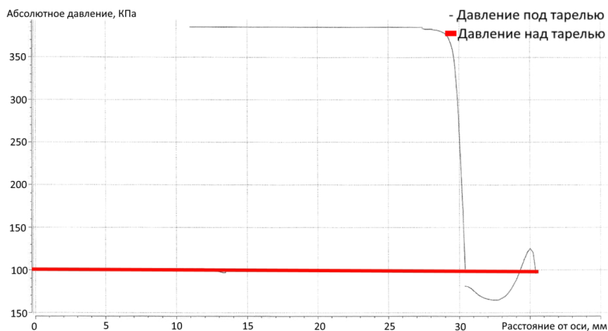
Рис. 8. График распределения давлений ( h=0,5 мм) для геометрии с уступом глубиной 2 мм
