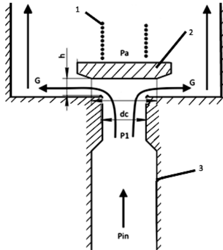
Рис. 1. Принципиальная схема предохранительного клапана
