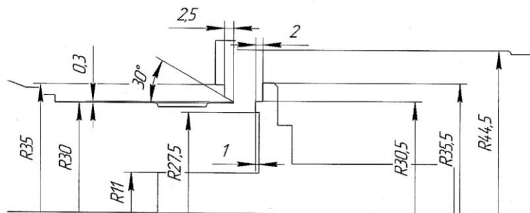
Рис. 5. Геометрия, с радиусом тарели с уступом глубиной 2 мм
