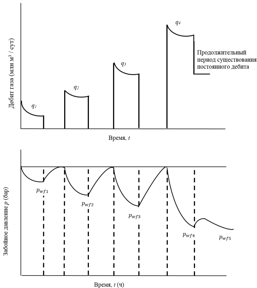
Рис. 2. Динамика давлений и дебитов в ходе типового исследования изохронным методом
