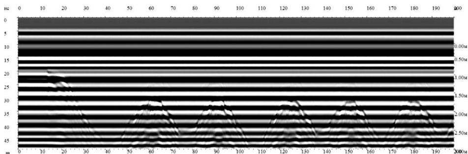
Рис. 2. Пример радарограммы движения человека за стеной
