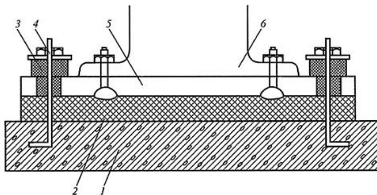
1 — фундамент; 2 — виброизолирующая прокладка; 3 — виброизолирующая втулка; 4 — анкерный болт с гайкой; 5 — плита; 6 — опорная конструкция силового агрегата Рис. 2. Установка оборудования через виброизолирующую прокладку
