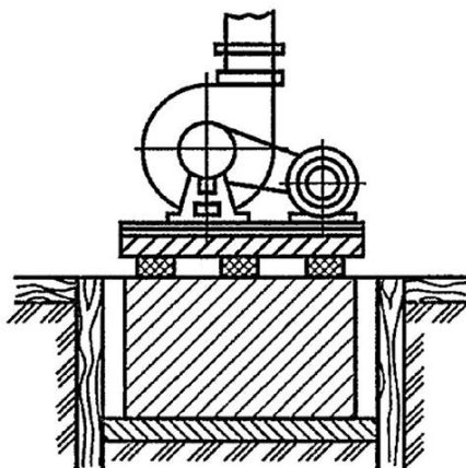
Рис. 1. Установка силового агрегата на вибропоглощающий массивный фундамент в грунте
