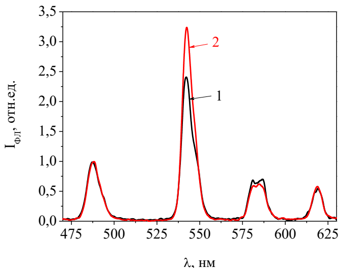
Рис. 1. Спектры ФЛ 0.005\text{ M Tb}^{3+} в воде (1) и 10\text{ M H}_2\text{SO}_4 (2). Спектры нормированы при \lambda = 488\text{ нм} . Спектрофлюориметр Fluorolog – 3, \Delta\lambda - 2\text{ нм}
