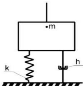
M – упругозакрепленная машина; K – общий коэффициент жесткости пружин; h – коэффициент деформирования
